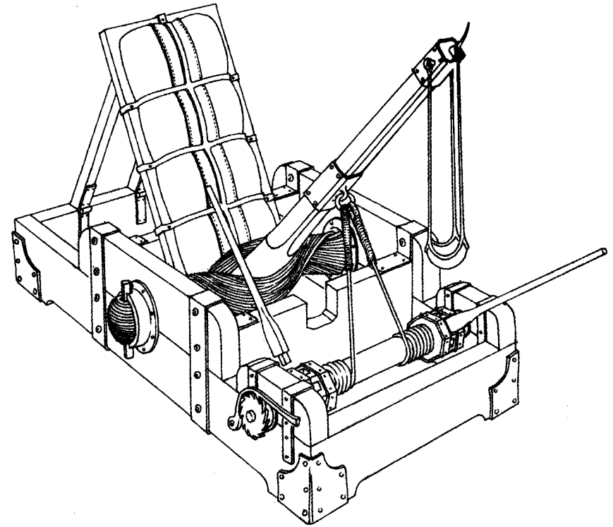
Рис. 66. Онагр по описанию Аммиана Марцеллина. Рис. И. В. Кирсанова.
