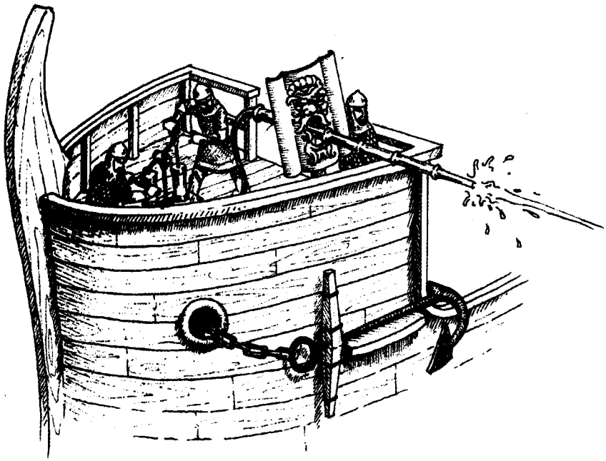
Рис. 121. Сифон для метания «греческого огня». По: Beffeyte R. L'art de la guerre au Moyen Âge. Rennes, 2005. P. 42. Рис. И. В. Кирсанова.
