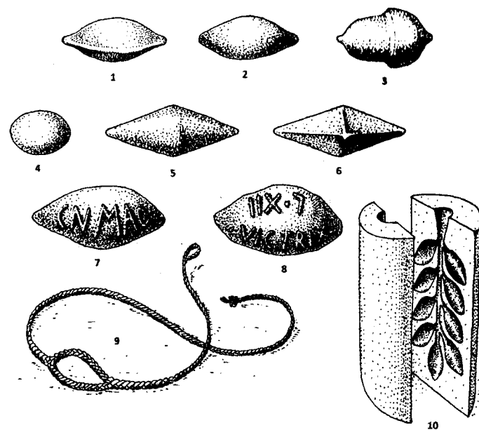
Рис. 47. 1–6 — наиболее распространенная форма пуль для пращей; 7 — свинцовая пуля, обнаруженная в Испании; датируется временем войны Помпея против Сертория; надпись: CN(eus Pompeus) MAC(nus); 8 — свинцовая пуля, обнаруженная в Перудже; 9 — праща из пеньки; такие пращи еще и сегодня делают на Балеарских островах; 10 — Реконструкция формы для отлива свинцовых пуль для пращей. По: Cascarino G. L'esercito Romano. Armamento e organizzazione. Vol. II: Da Augusto ai Severi. Rimini, 2008. P. 90–93. Рис. И. В. Кирсанова.
