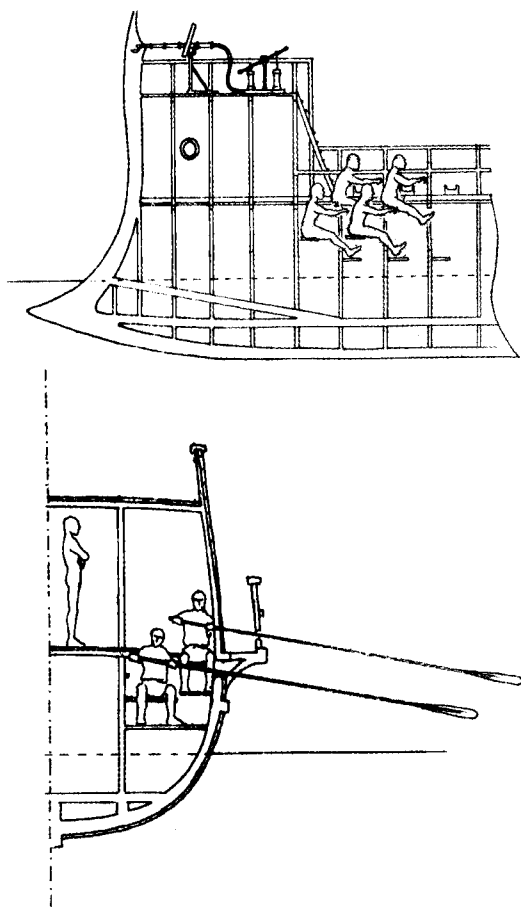
Рис. 117, 118. Предполагаемая схема внутреннего устройства дромона.
