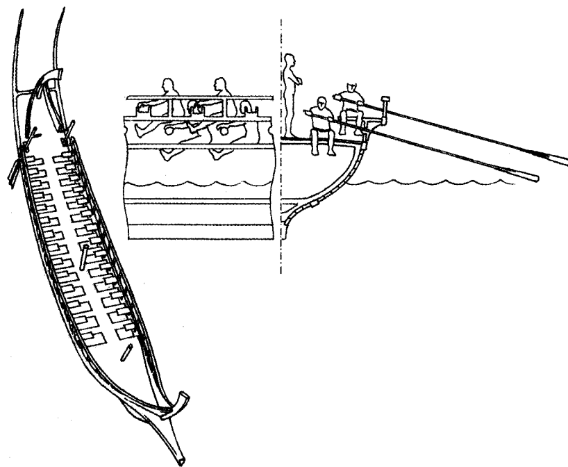
Рис. 119. Византийский дромон IX–X вв.
