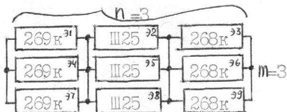
Рис.2. Поэлементное резервирование системы 6КС (альтернативный, предлагаемый вариант).
