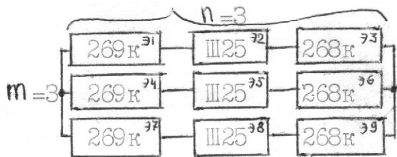
Рис.1. Общее резервирование системы 6КС (существующий вариант).
