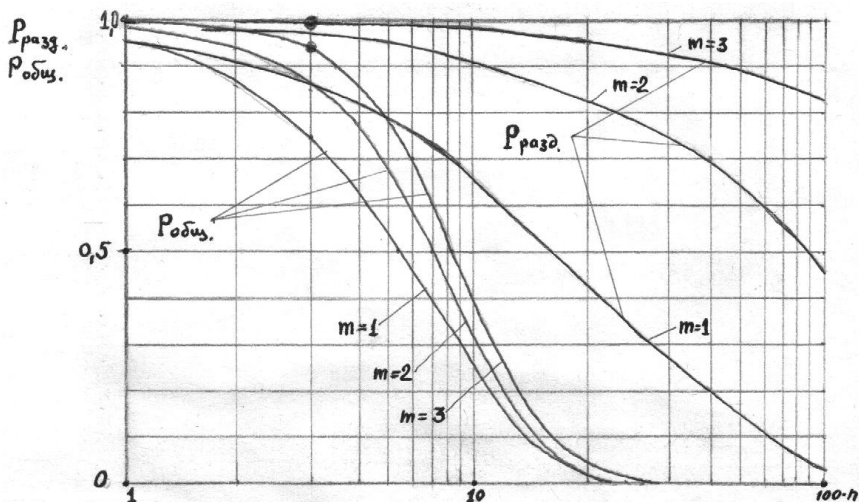
Рис.4.33. Зависимость вероятности безотказной работы от числа элементов системы при различных видах резервирования.
