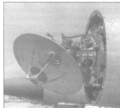
Редкий снимок - антенна РЛС «Орел».
