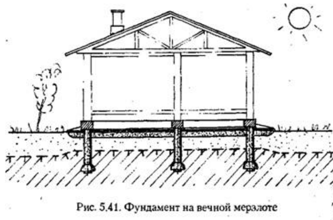
Рис. 6. Схема строительства дома на вечной мерзлоте
