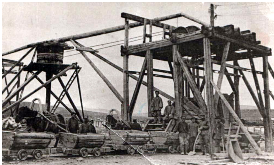
Рис. 1. Золотопромывальная машина
