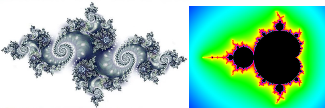
Рис. 4. Множества Жюлиа (слева) и Мандельброта (справа)
